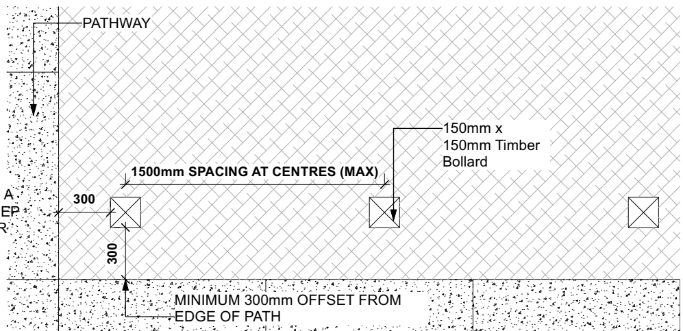
SETOUT PLAN
